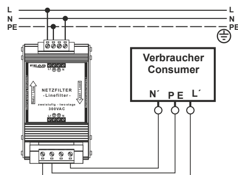
Anschlußbeispiel
