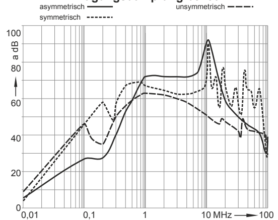
Einfügungsdämpfung bei 50 Ω
