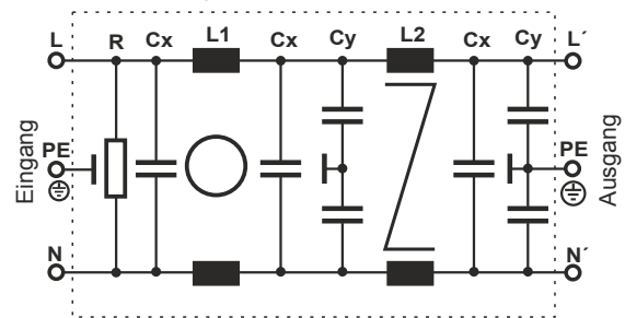
Typisches Schaltbild
